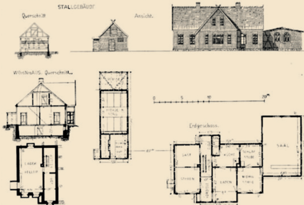
Fig. 196–200. Kruggehöft nebst Kaufmannsladen zu Borkow. Architekt: Fr. Wagner in Rostock.
